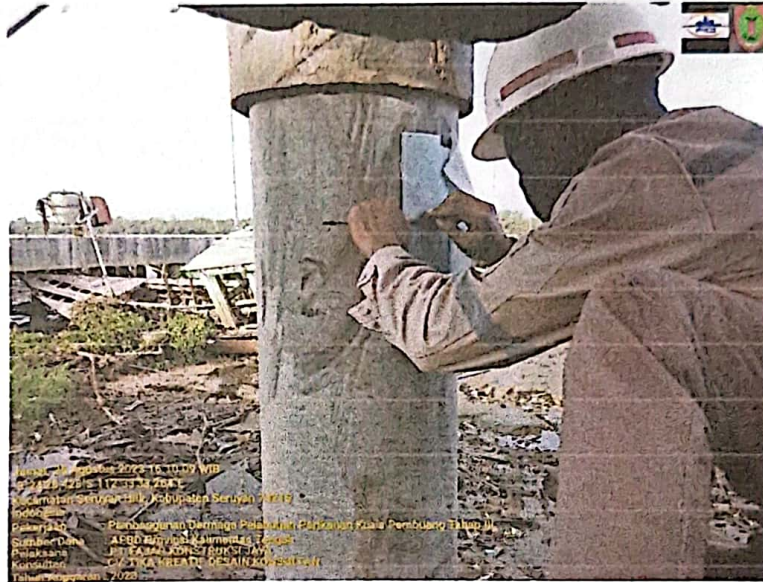
TES KALENDERING PADA TIANG SPON PILE
