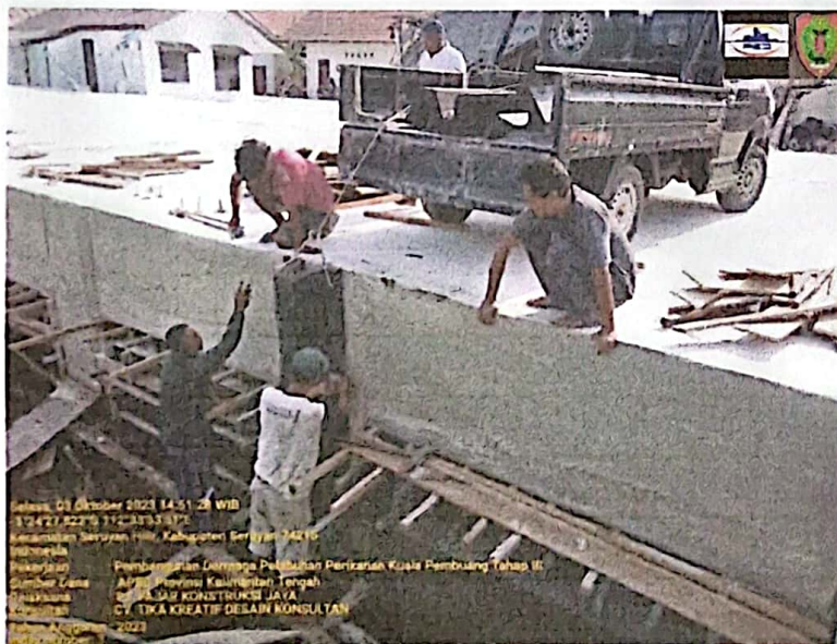
PEKERJAAN PEMASANGAN FENDER
