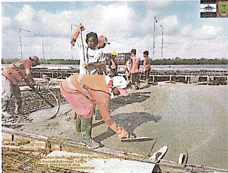
PEKERJAAN PENGECORAN LANTAI DERMAGA
