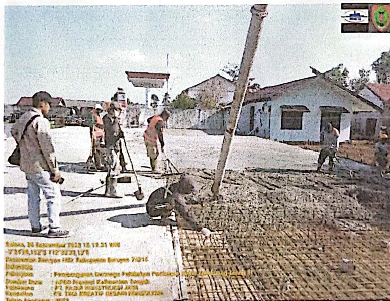
PEKERJAAN PENGECORAN SELASAR DERMAGA
